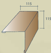
13 Vidinis kampas ilgis 2000 mm
