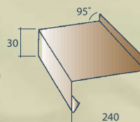
18 Palangė 240 ilgis 2000 mm
