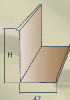
25 PZ profilis aukštis 50 ir 100 mm storis 1,0 ir 1,2 mm
