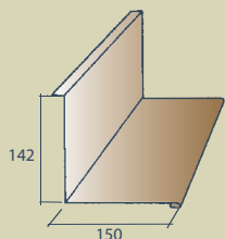
9 Stogo - sienos kampas ilgis 2000 mm
