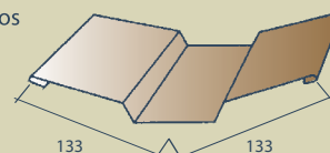
15 Palangė 90 ilgis 2000 mm
