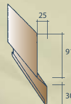
19 Cokolio detalė ilgis 2000 mm
