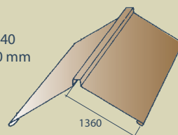
4 Antgalis apvaliam kraigui
