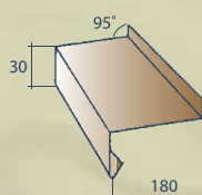
17 Palangė 180 ilgis 2000 mm
