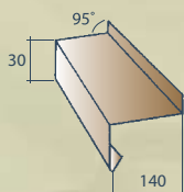
16 Palangė 140 ilgis 2000 mm
