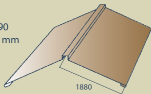
3 Apvalus kraigas ilgis 1980 mm
