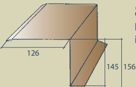
7 Vėjalentė 145 ilgis 2000 mm
