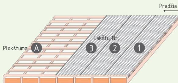
2 paveikslėlis - montavimo schema.
